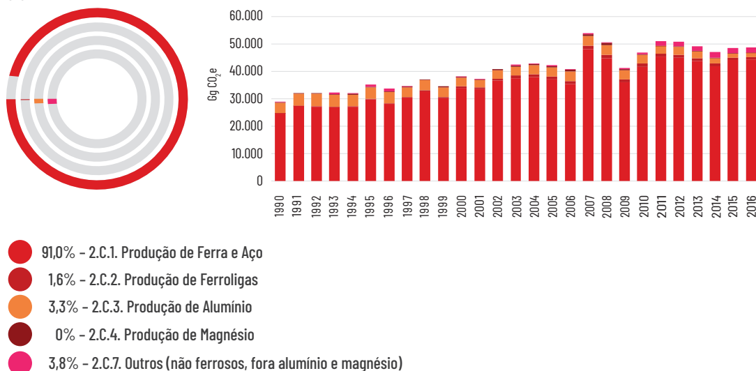
Figura 2.22 Emissões da Indústria Metalúrgica (2.C), em \text{CO}_2\text{e} , por categoria, de 1990 a 2016.
